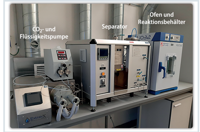
Bild 3. Der Reaktor bei Centexbel mit Flüssigkeitspumpe, Reaktionsraum im Ofen und einem Separator zur Trennung der Kontamination.
