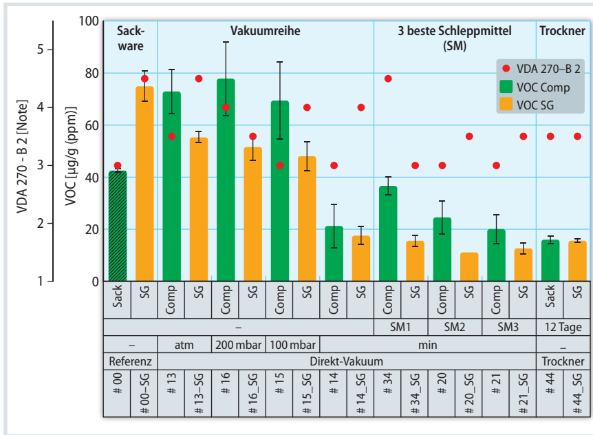
Bild 1. Ermittelte Kennwerte für die VOC-Emissionen und Geruch nach der Behandlung im Stripping-Prozess. (Comp = nach Extrusion, SG = nach Spritzgießen) Quelle: Fraunhofer ICT; Grafik: © Hanser
